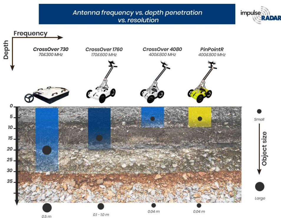
شکل ۲-۱- فرکانس آنتن در مقابل میزان عمق نفوذ و رزولوشن.
