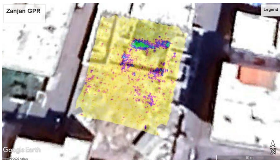
شکل ۳-۴- تصویری از نمونه خروجی در نرم افزار Geolitic؛ نمایش برشی از مدل سه بعدی آنتن ۴۰۰ مگاهرتز بر روی تصویر ماهواره ای.
